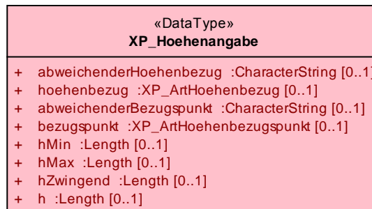
Abbildung 7: XPlanung Datenstruktur zur Spezifikation einer Höhenangabe (UML-Modell)
