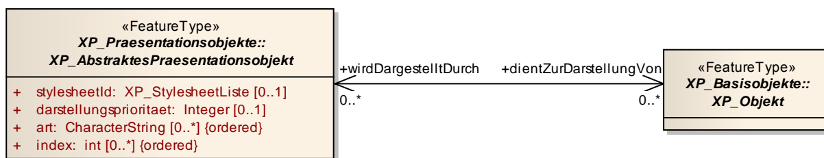
Abbildung 8: XPlanung Basisklasse für Präsentationsobjekte (UML-Modell)
