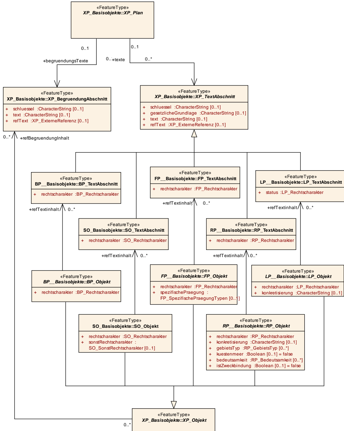
Abbildung 4: Textliche formulierte Planaussagen und Plan-Begründung (UML-Modell)
