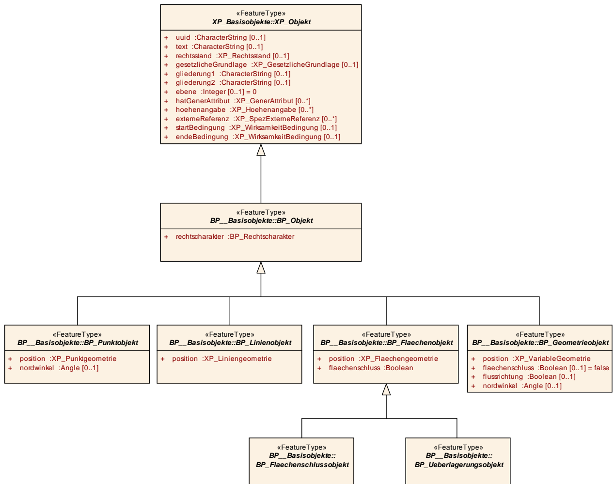
Abbildung 6: Raumbezug der Fachobjekte des BPlans (UML-Modell)
